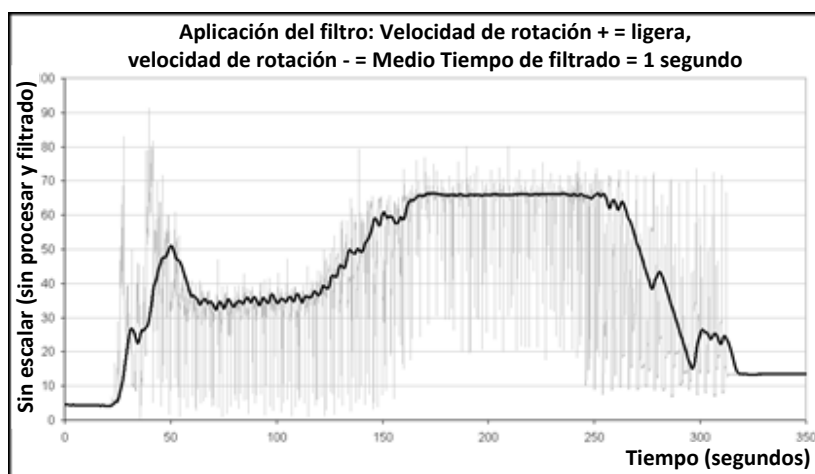
Ilustración 8: Filtrado de la señal sin escalar/sin procesar (1)
