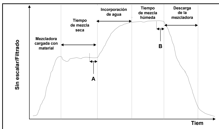
Ilustración 6: Curva de humedad normal
