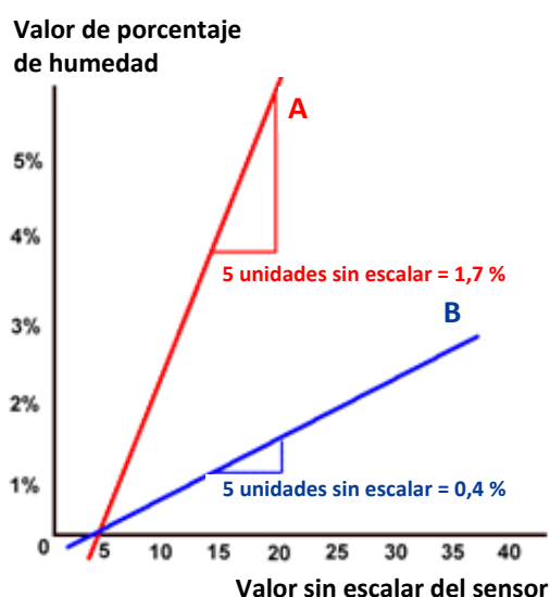
Ilustración 10: Relación de los valores Sin escalar respecto a la humedad
