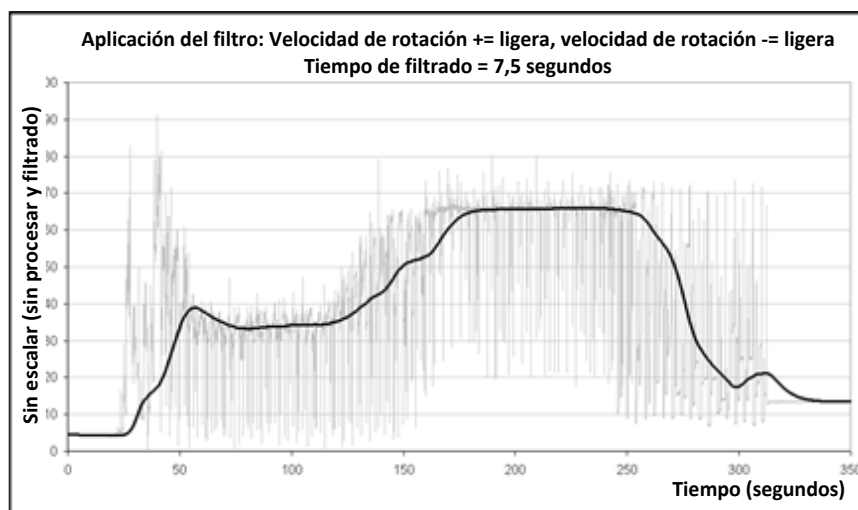
Ilustración 9: Filtrado de la señal SIN PROCESAR (2)
