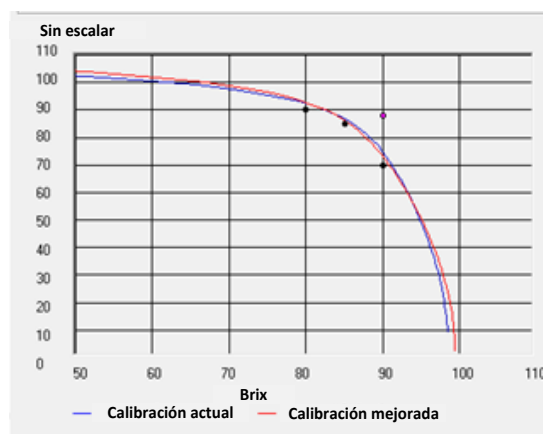
Ilustración 23: Ejemplo de una mala calibración de Brix
