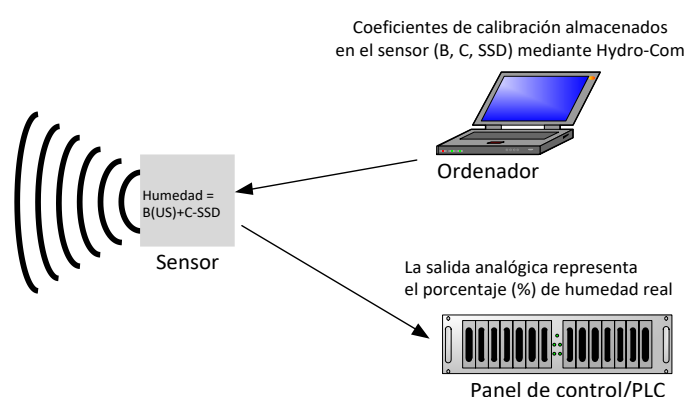
Ilustración 16: Calibración dentro del sensor
