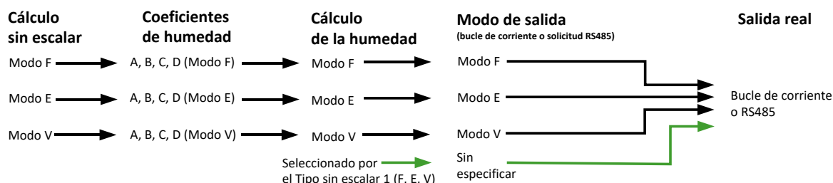
Ilustración 12: Ninguna selección de salida especificada
