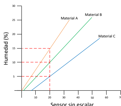
Ilustración 14: Calibraciones para 3 materiales diferentes
