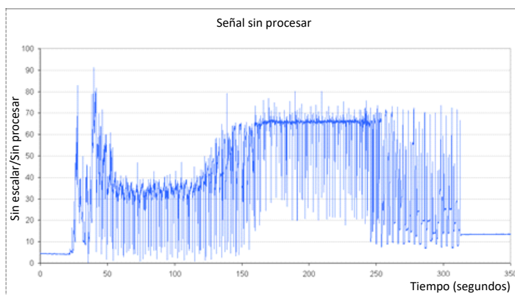
Ilustración 7: Gráfico que muestra la señal sin procesar durante el ciclo de mezcla
