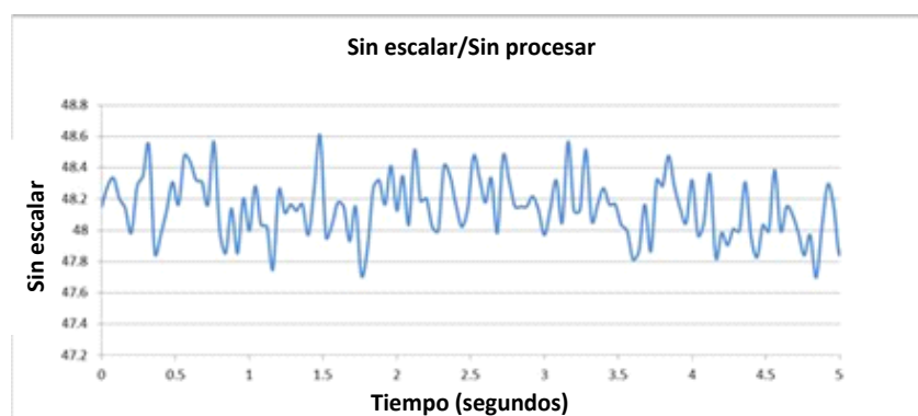
Ilustración 4: Rastro de humedad sin escalar/sin procesar en el material que fluye
