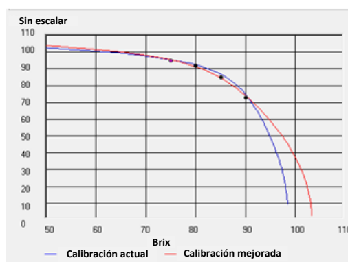
Ilustración 22: Ejemplo de una buena calibración de Brix
