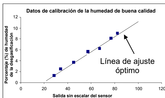
Ilustración 18: ejemplo de una buena calibración del material
