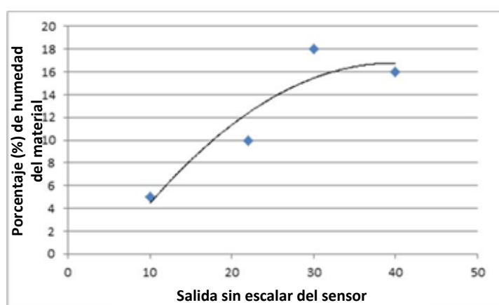
Ilustración 21: Ejemplo de una mala calibración cuadrática
