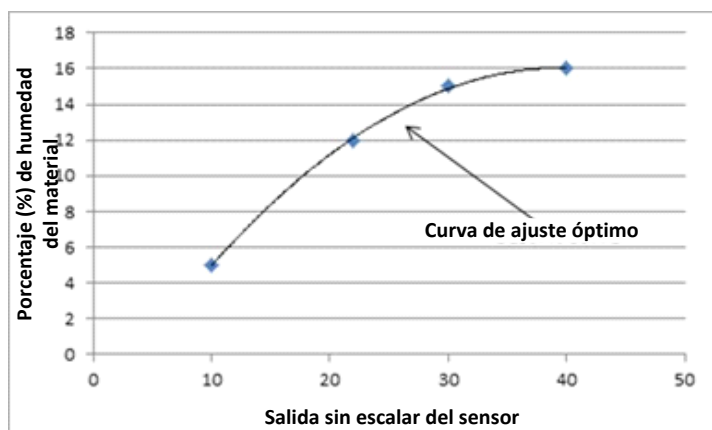
Ilustración 20: Ejemplo de una buena calibración cuadrática
