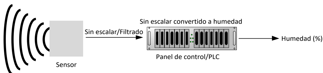
Ilustración 17: Calibración dentro del sistema de control
