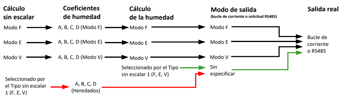
Ilustración 13: Selección de salida antigua
