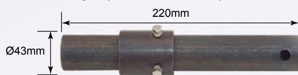
Manguito y abrazadera de montaje de extensión
